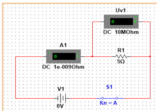
Рис. 9. Дослідження закону Ома для ділянки кола
