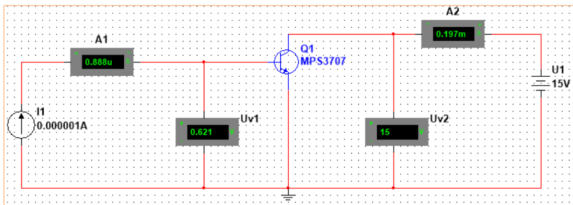
Рис. 30. Схема для зняття V_{AX} біполярного транзистора в Multisim
