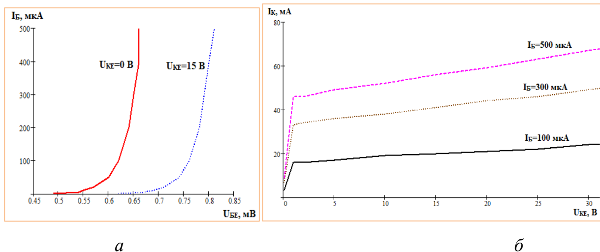
Рис. 31. Вольт-амперні характеристики біполярного транзистора, побудовані в Mathcad: а – вхідні, б – вихідні
