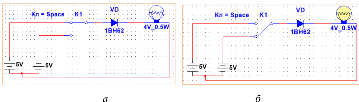
Рис. 21. Дослідження принципу дії напівпровідникового діода в колі постійного струму : а – лампочка не світиться, б – лампочка світиться
