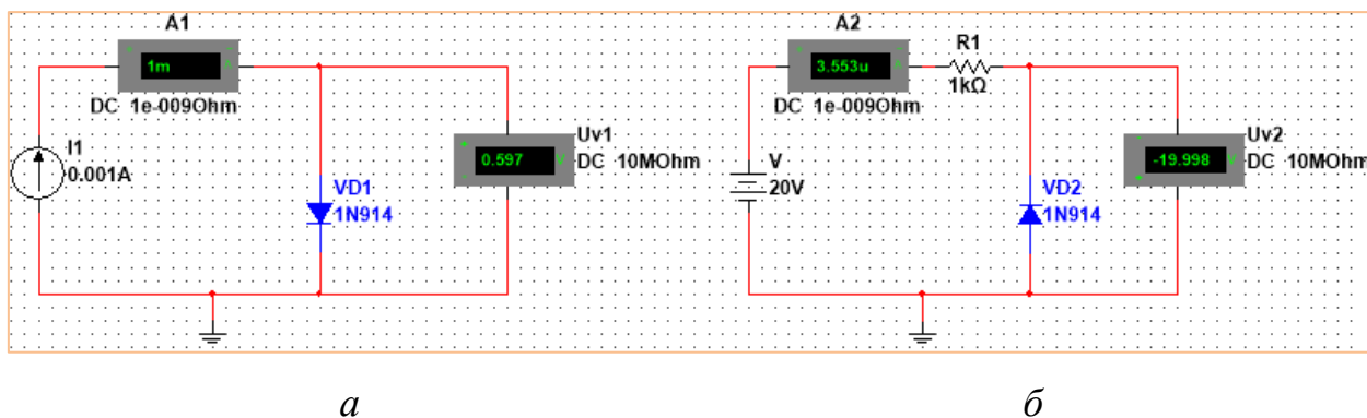
Рис. 19. Схеми для зняття VAX діода 1N914: a – пряме включення, b – зворотне включення
